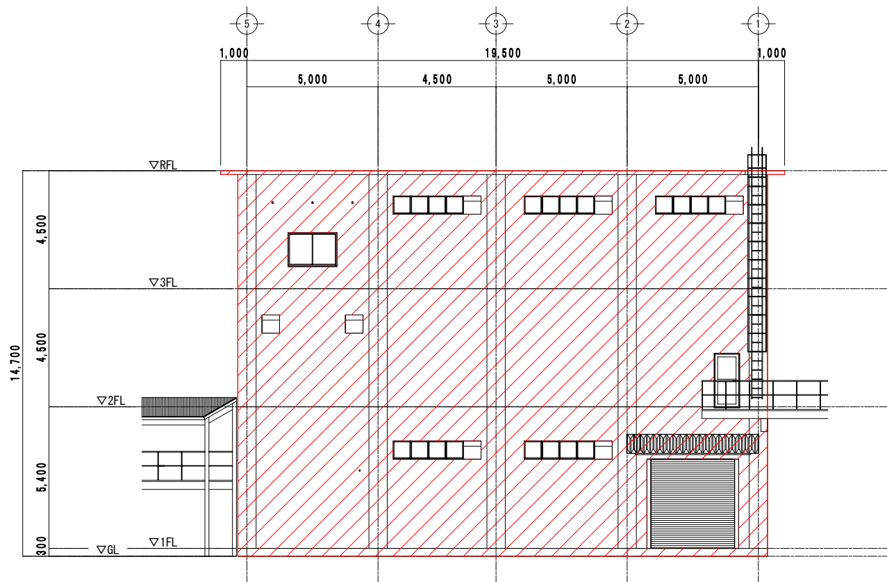
北側立面図
