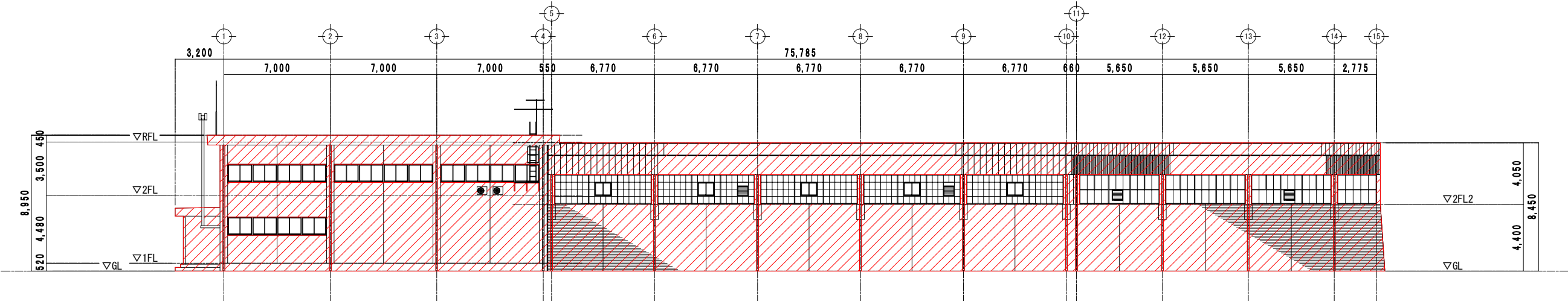
北側立面図
