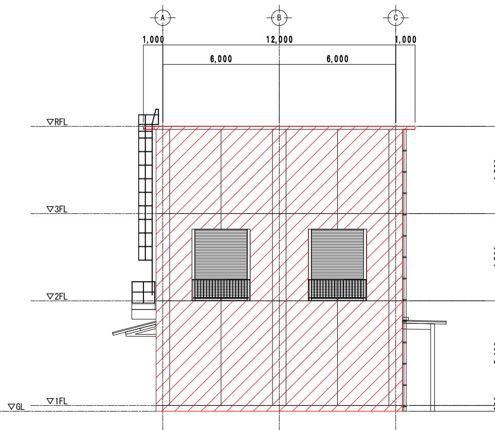
西側立面図
