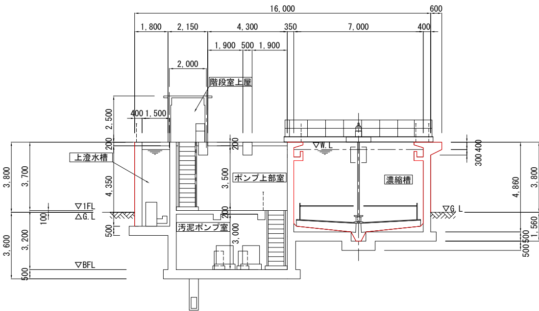
B-B断面図
