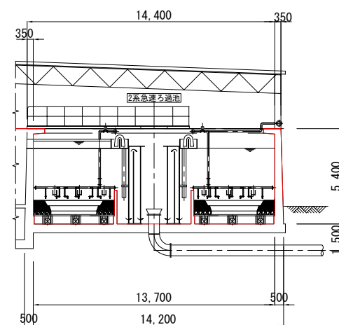
B-B断面図
