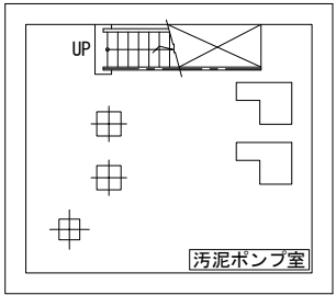
排泥池・濃縮槽 平面図 (最下部)
