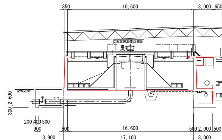
C-C断面図
