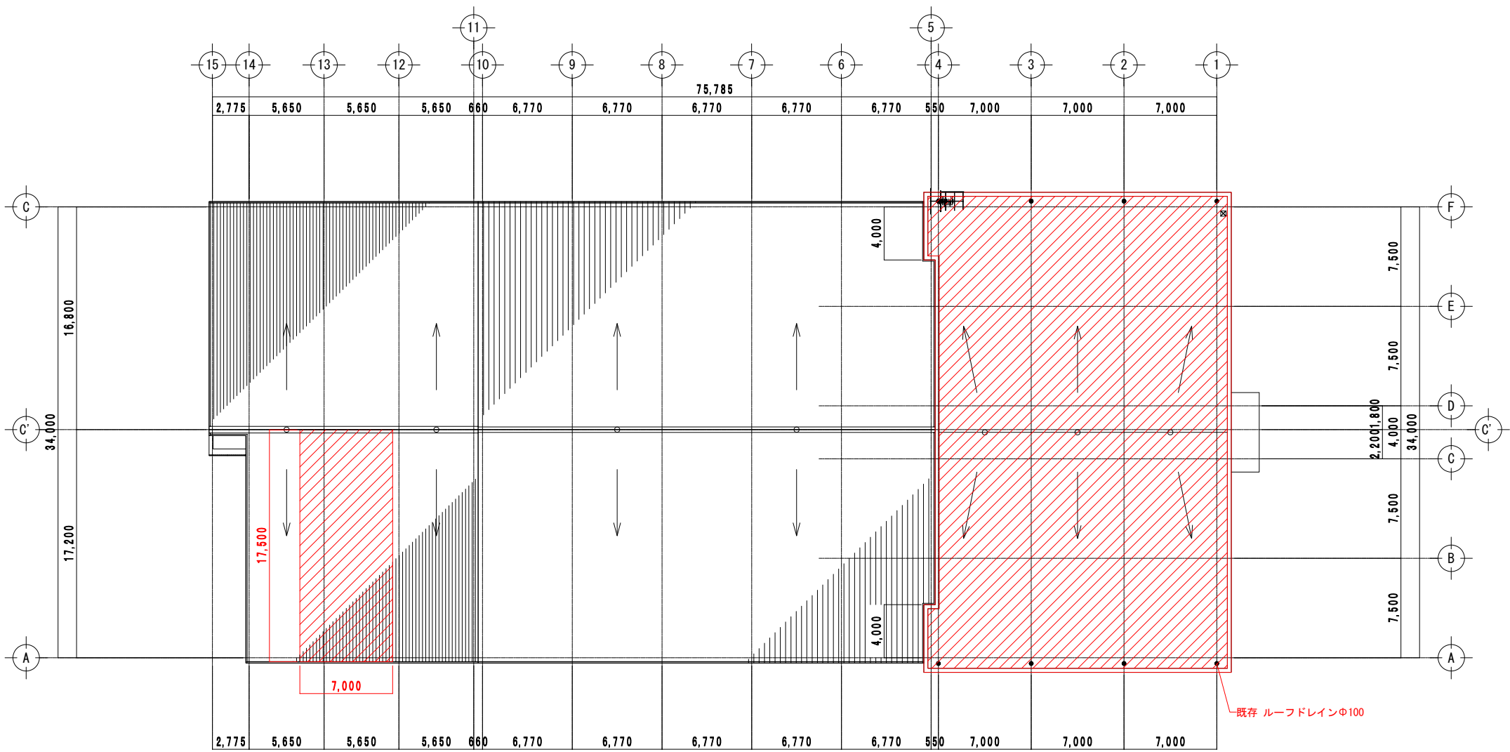
屋根伏図
