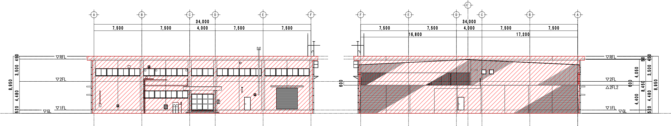
東側立面図
