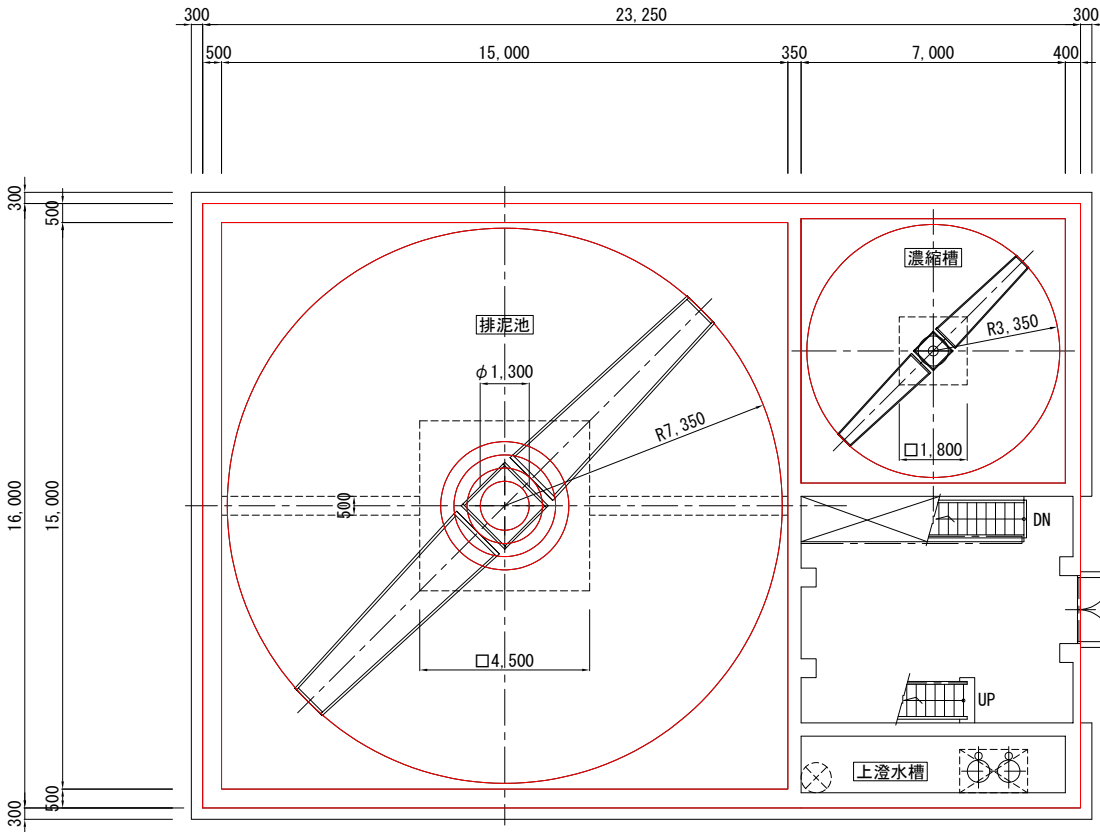
排泥池・濃縮槽 平面図 (下部)
