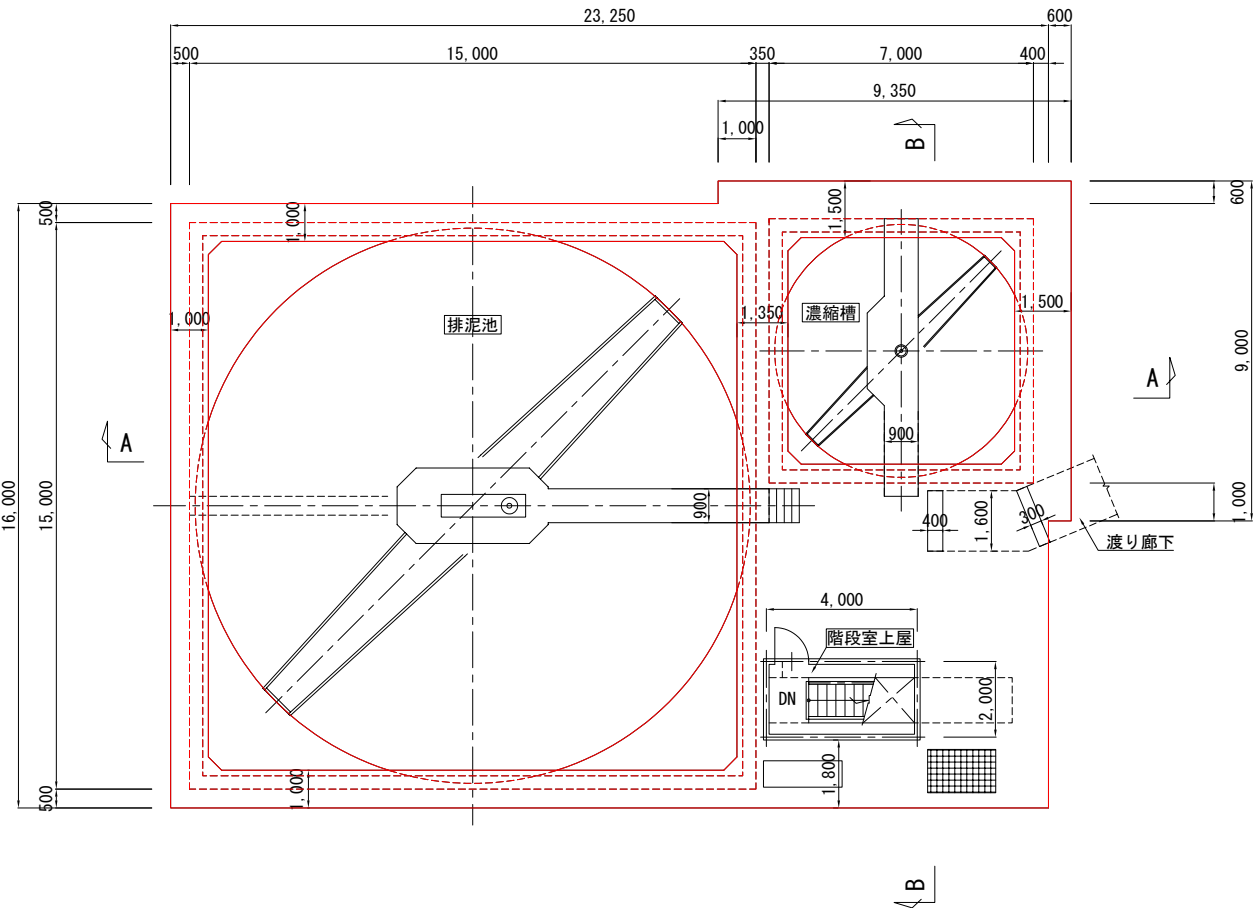
排泥池・濃縮槽 平面図 (上部)
