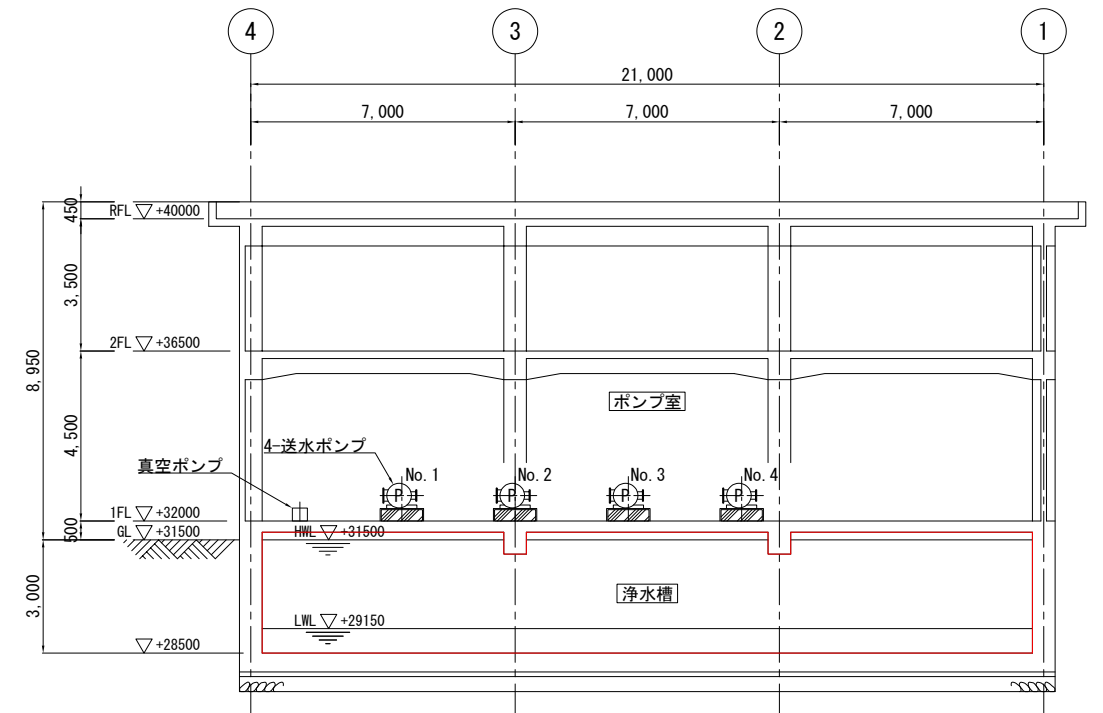
管理棟 断面図
