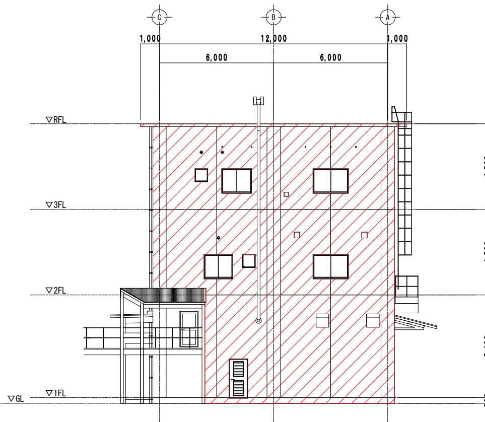
東側立面図
