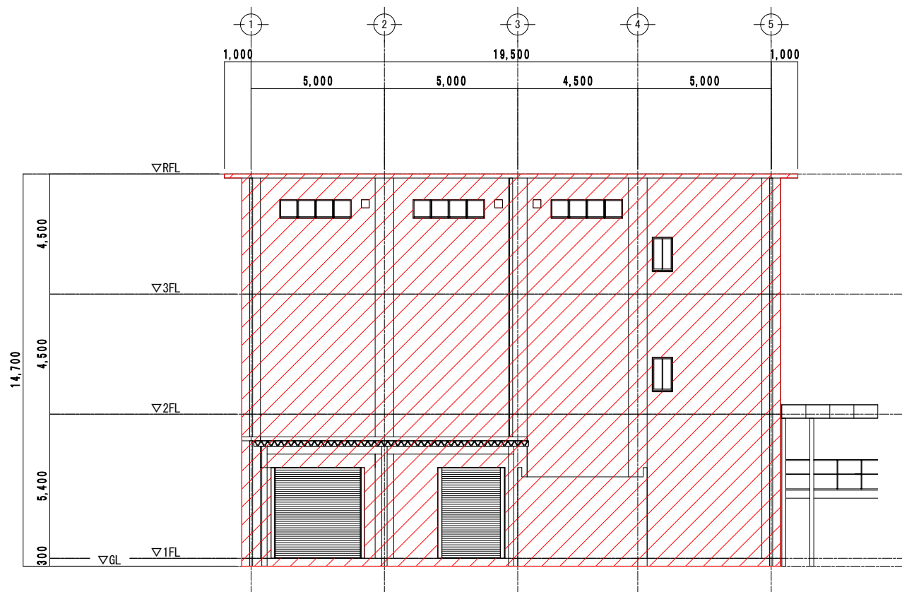
南側立面図
