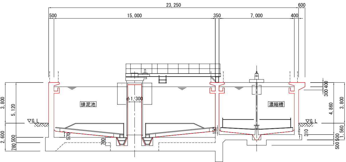
A-A断面図
