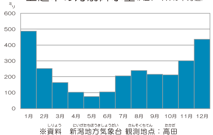
じょうえつし つきべつこうすいりょう へいぎんち 上越市の月別降水量 (H27～R1の平均値)
